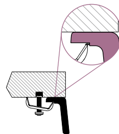
Spodní uložení montáž s příchýtkami
