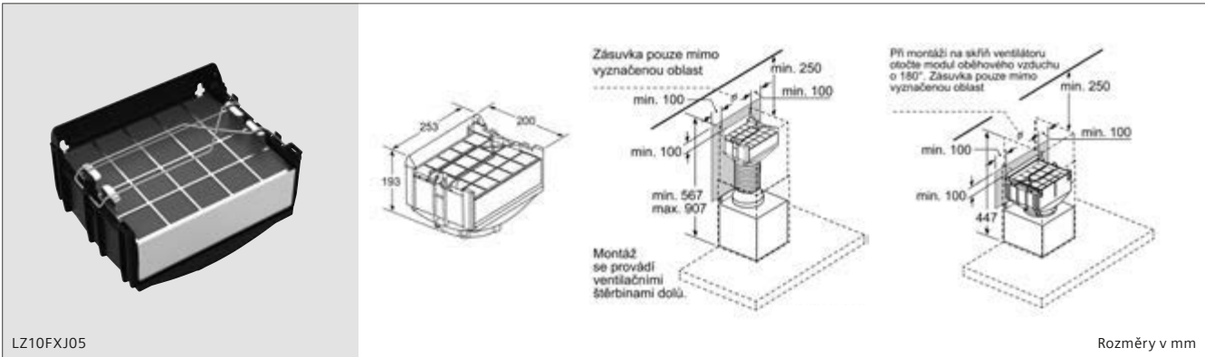
Regenerační longLife cleanAir Plus montážní sada pro výsuvné odsavače par
