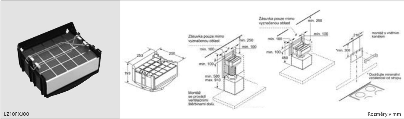
Montáž snižovacího rámečku pro výsuvný odsavač par, 90 cm
