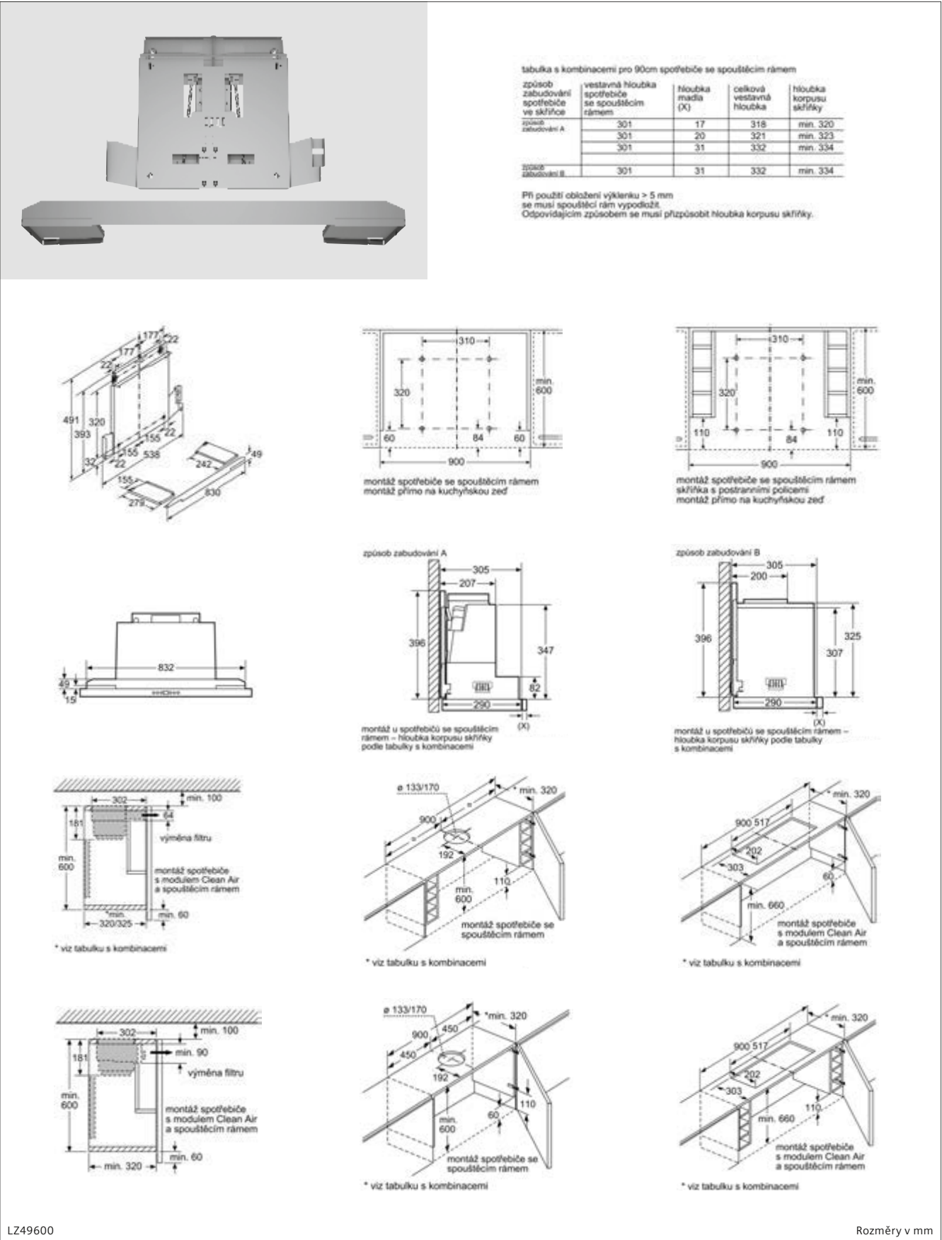
Montage Absenrahmen-Umluftmodul für Flachschrilmhauben, 90 cm
