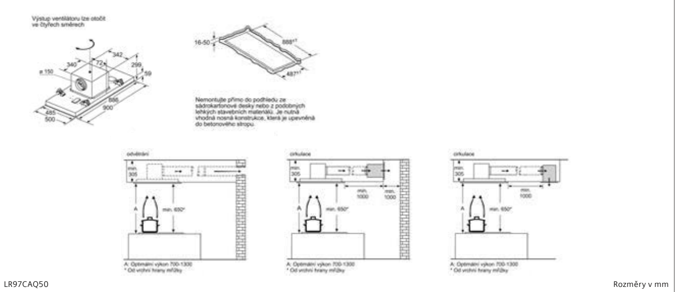
Stropní odsavač par, 90 cm
