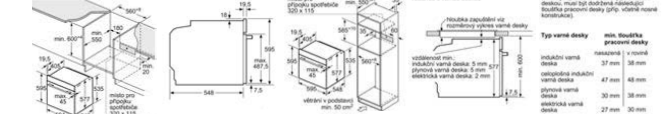
Kombinovaná trouba s mikrovlnami
